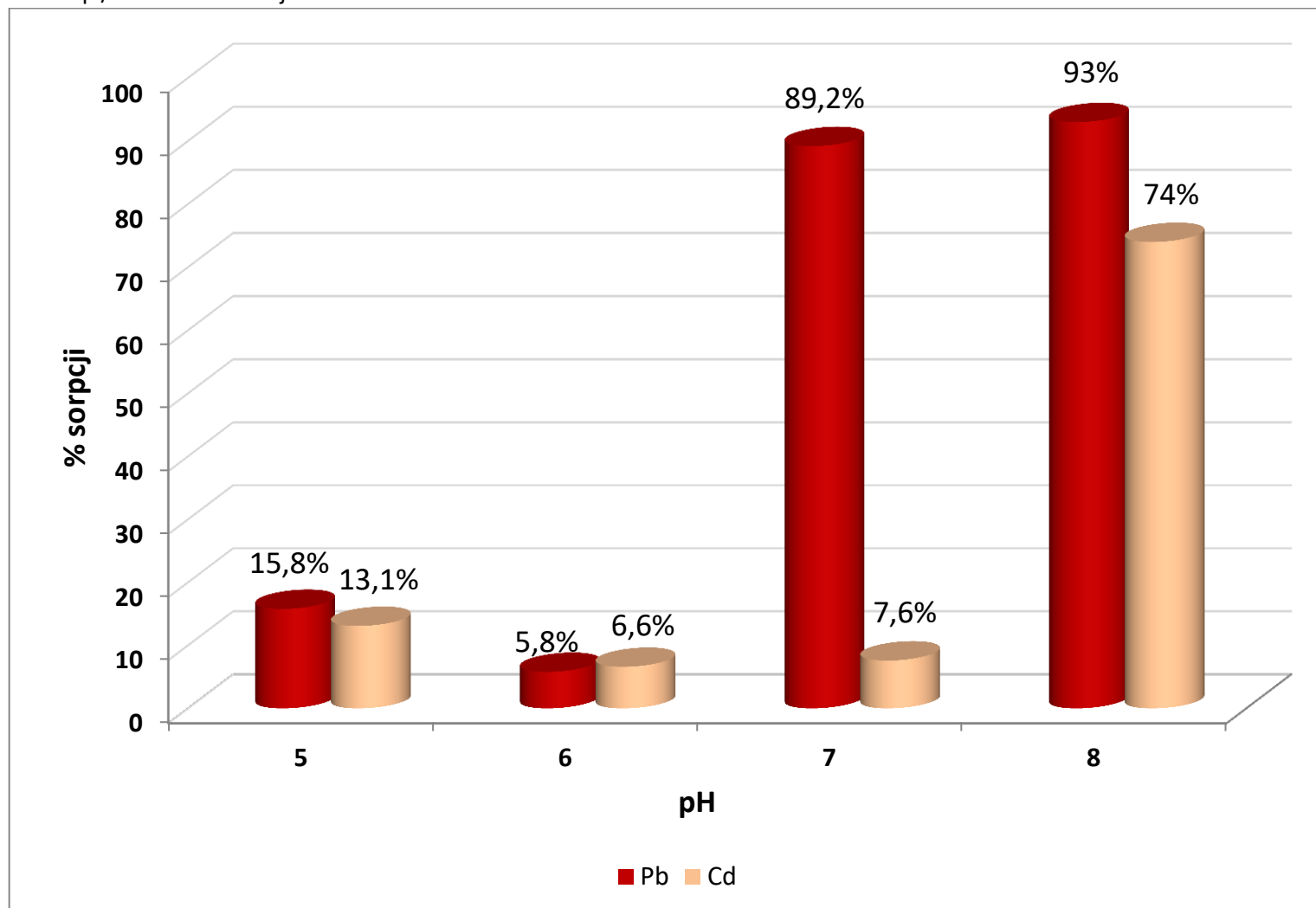
Wykres 1 Wpływ pH na procent sorpcji wybranych jonów metali na tkaninie poliestrowej wybarwionej 5-[( E )-(3-hydroksyfenylo)diazenylo]-8-hydroksy-2-metylochinolimą. Pomiar zawartości jonów metali wykonano techniką ICP-OES. Oprac. dr Barbara Feist
